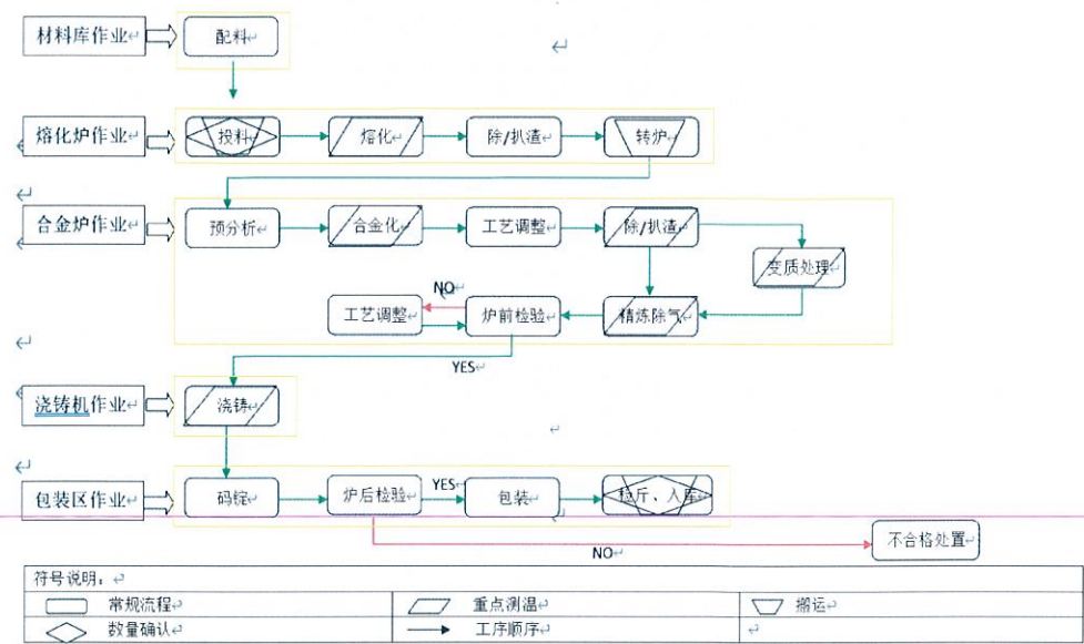
图 2.3.1：再生铝锭生产加工过程
