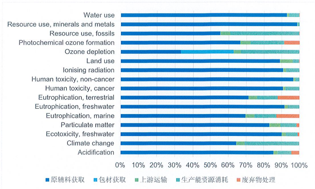
图 5.1.1 1t 再生铝锭分活动环境影响贡献比例
