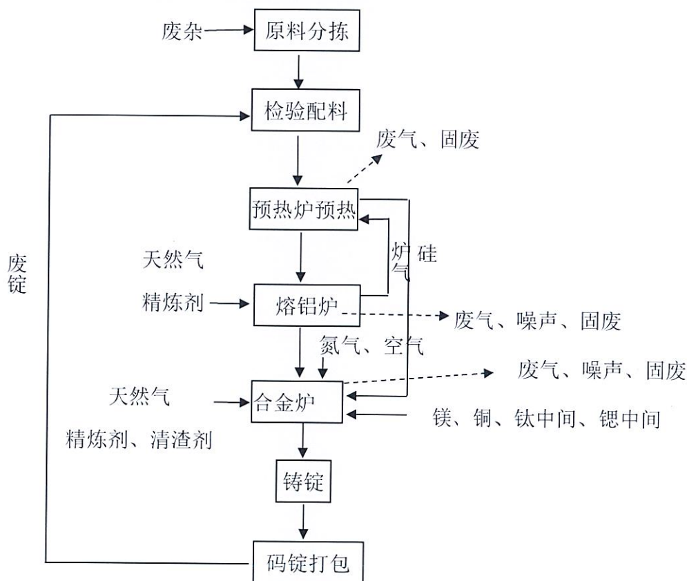
图 2.3.1：100%再生铸造铝合金锭生产加工过程
