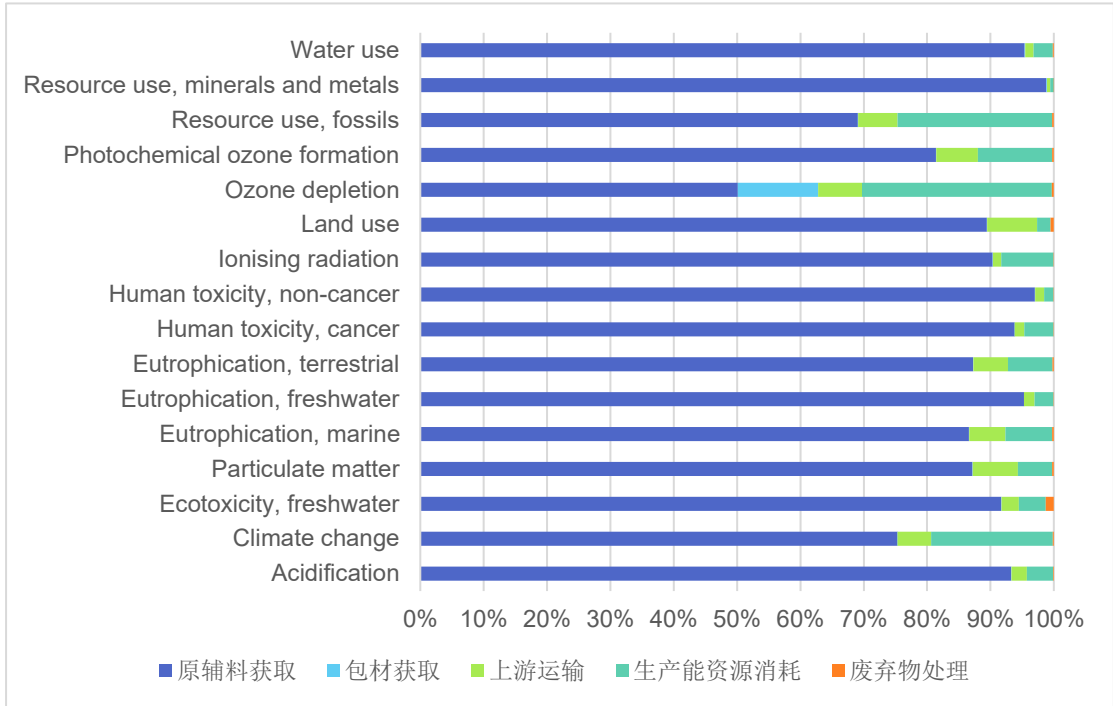
图 5.1.1 1t 铸造再生铝合金锭分活动环境影响贡献比例
